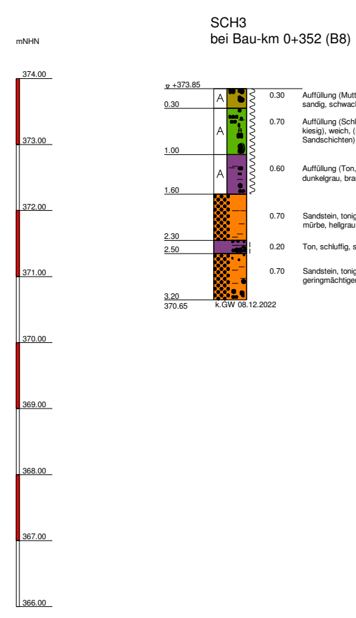
Schurfprofil Maßstab 1: 2,5
